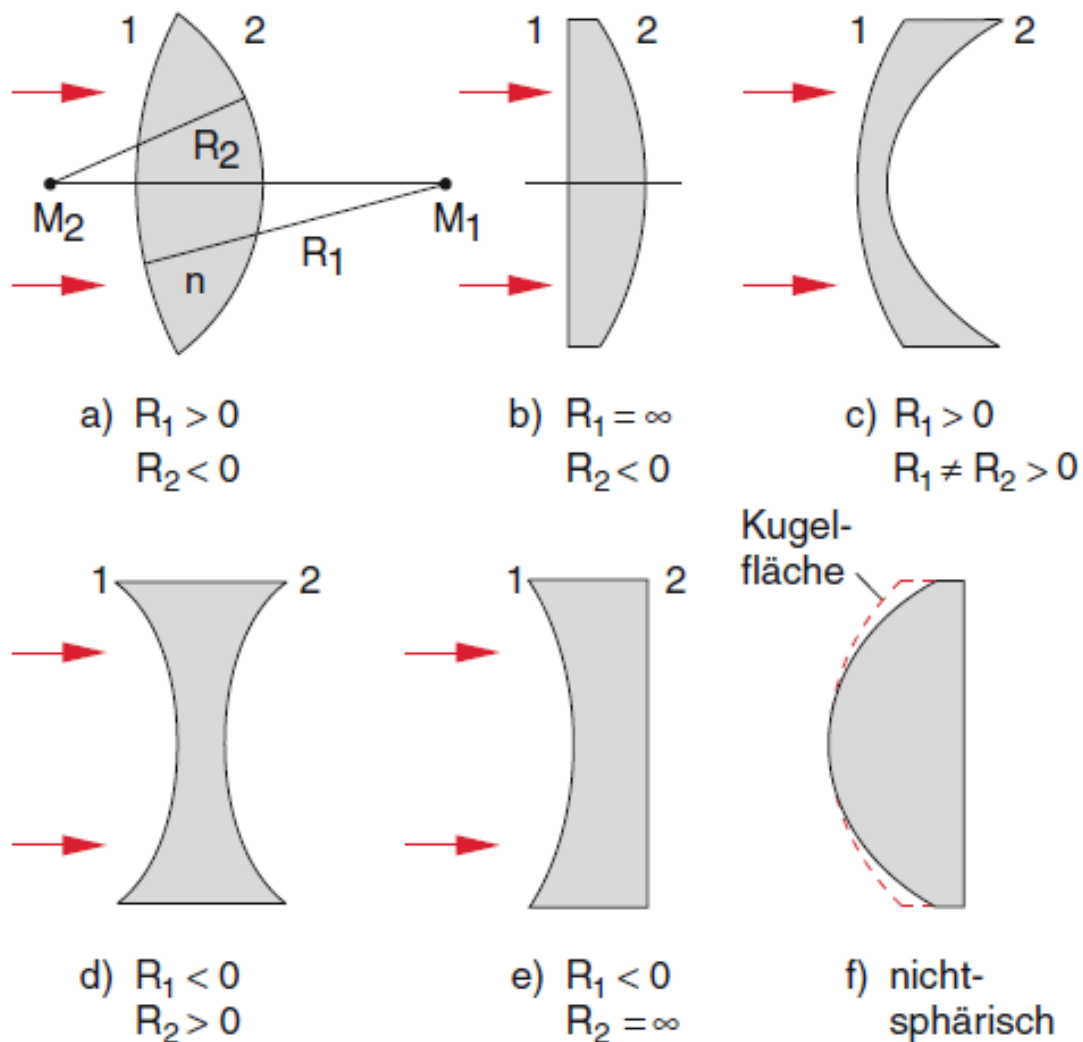
Abbildung 9.25 Beispiele für verschiedene Linsenformen. a konvex-konvex = bikonvex, b plan-konvex, c konvex-konkav, d bikonkav, e konkav-plan, f nichtsphärische Linse
