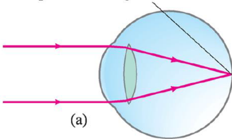
Brennpunkt von Augenlinse und Hornhaut
